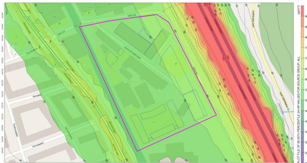
Figur 7. Nuvarande situation 2013/2015, beräknade halter av kvävedioxid som dygnsmedelvärden. Planområdet markeras med lila linje och föreslagna byggnader med blå
