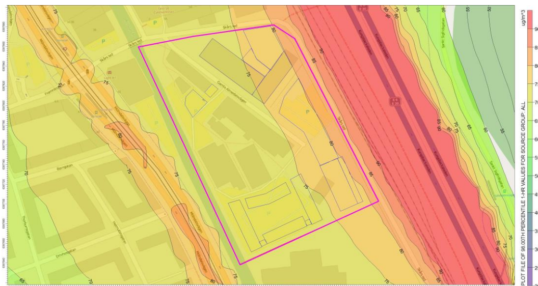
Figur 10. Nuvarande situation 2013/2015, beräknade halter av kvävedioxid som timmedelvärden. Planområdet markeras med lila linje och föreslagna byggnader med blå
