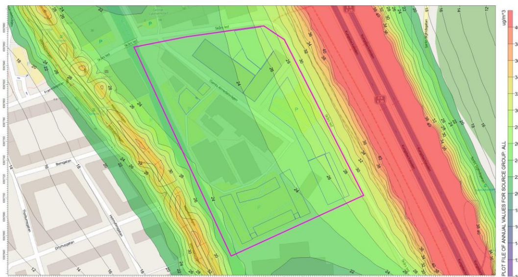
Figur 4. Nuvarande situation 2013/2015, beräknade halter av kvävedioxid som årsmedelvärden. Planområdet markeras med lila linje och föreslagna byggnader med blå
