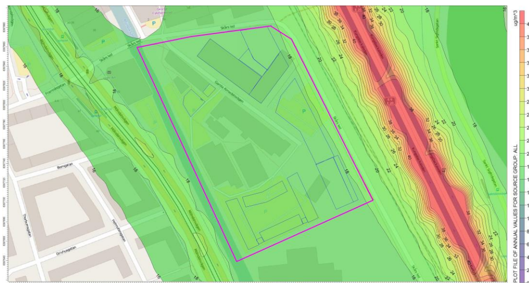
Figur 14. Framtida scenario 2020, beräknade halter av partiklar (PM 10 ) som årsmedelvärden. Planområdet markeras med lila linje och föreslagna byggnader med blå
