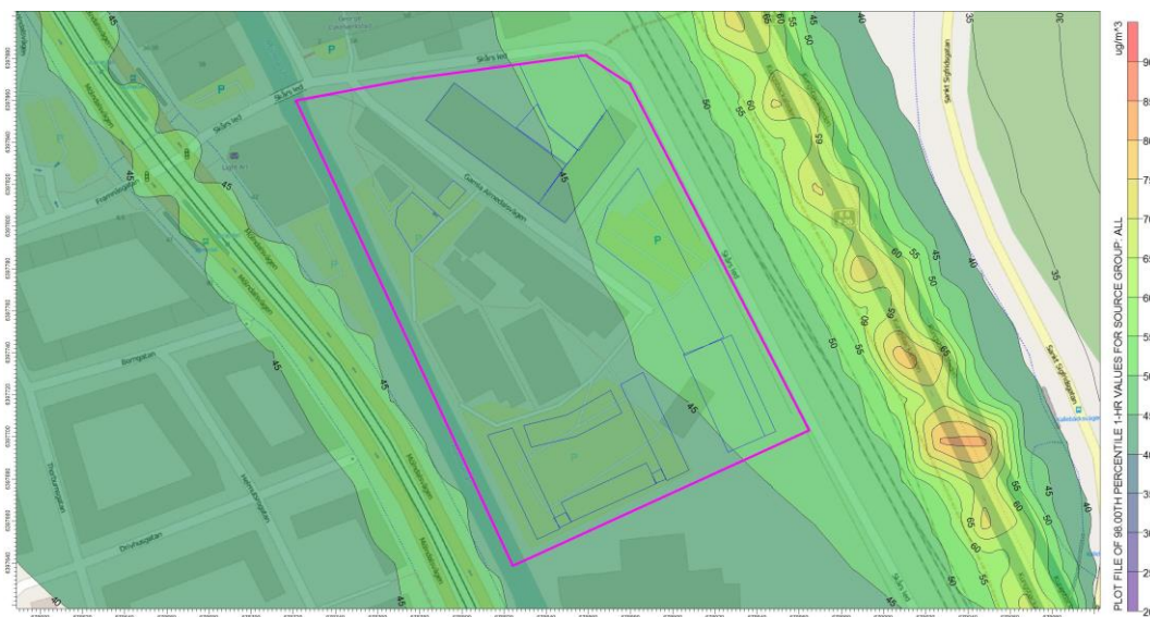
Figur 12. Framtida scenario 2030, beräknade halter av kvävedioxid som timmedelvärden. Planområdet markeras med lila linje och föreslagna byggnader med blå
