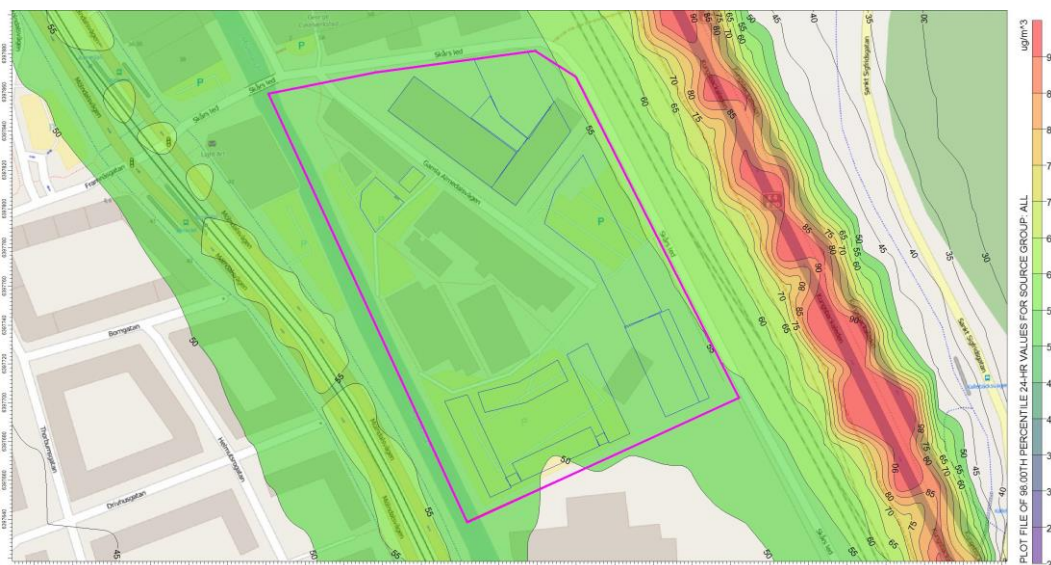
Figur 8. Framtida scenario 2020, beräknade halter av kvävedioxid som dygnsmedelvärden. Planområdet markeras med lila linje och föreslagna byggnader med blå
