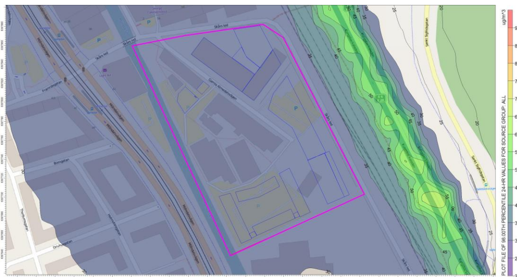
Figur 9. Framtida scenario 2030, beräknade halter av kvävedioxid som dygnsmedelvärden. Planområdet markeras med lila linje och föreslagna byggnader med blå
