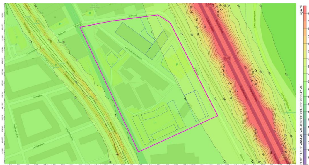
Figur 13. Nuvarande situation 2013/2015, beräknade halter av partiklar (PM 10 ) som årsmedelvärden. Planområdet markeras med lila linje och föreslagna byggnader med blå
