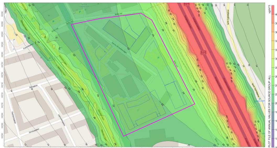
Figur 5. Framtida scenario 2020, beräknade halter av kvävedioxid som årsmedelvärden. Planområdet markeras med lila linje och föreslagna byggnader med blå
